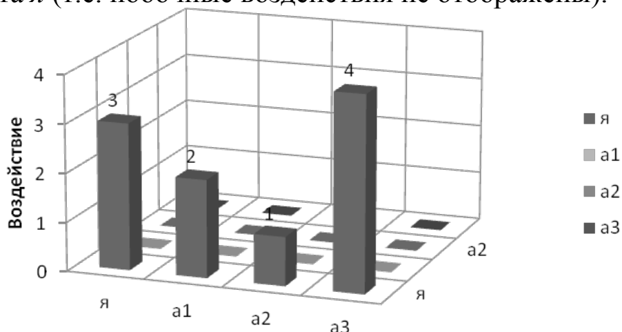
Рис. 2. Агенты я , a1 , a2 , a3 с различной степенью влияния
