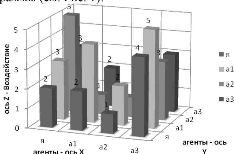
Рис. 1 Двумерная СПД с переменными: агенты и воздействия
