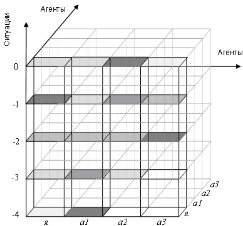
Рис. 3. Трёхмерная СПД с возможными вариантами динамики влиятельности агентов в интракультуре лица
